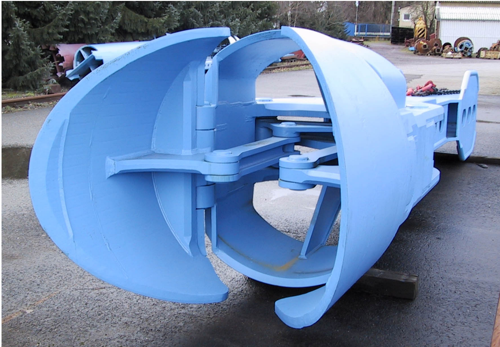
Volumengreifer VG 1380
